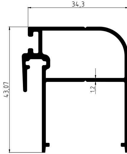
MS5103 0,580 Kg/Mt
