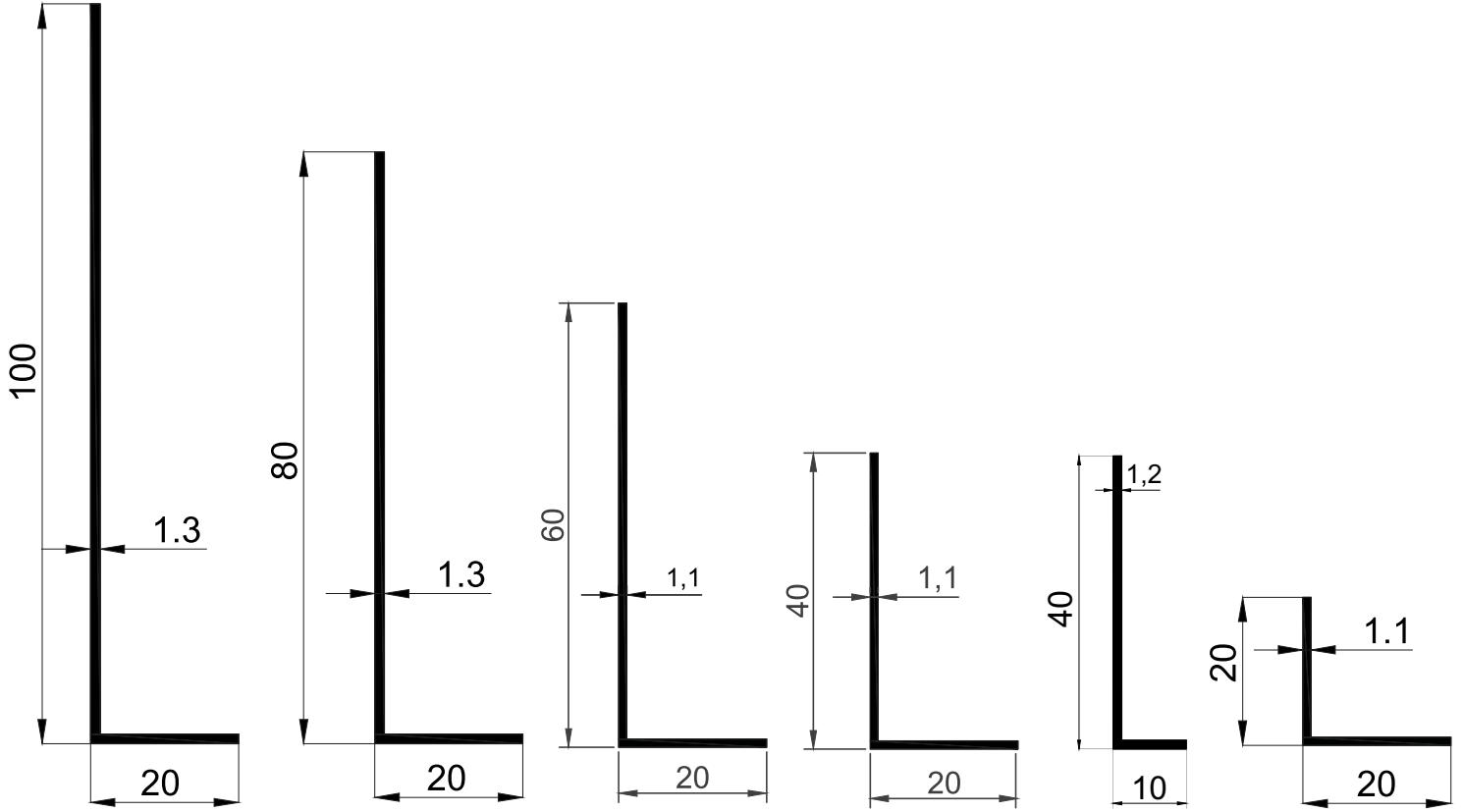
MS2001 0,428 Kg/Mt
