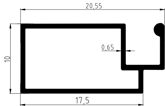
MS113 0,113 Kg/Mt
