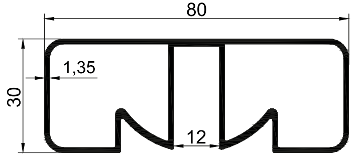
MS1093 0,910 Kg/Mt
