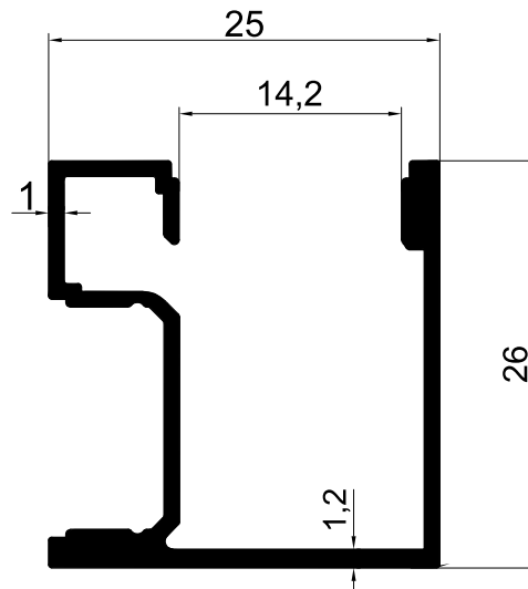
MS1050 0,305 Kg/Mt
