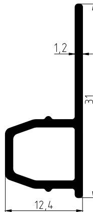
MS5100 0,195 Kg/Mt
