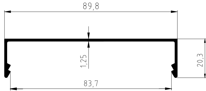
MSÖ41103 0,477 Kg/Mt
