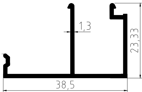
MS5507 0,344 Kg/Mt
