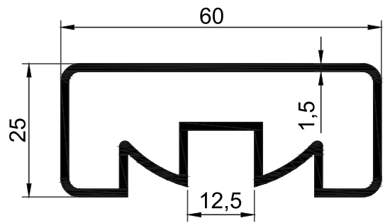
MS1079 0,740 Kg/Mt
