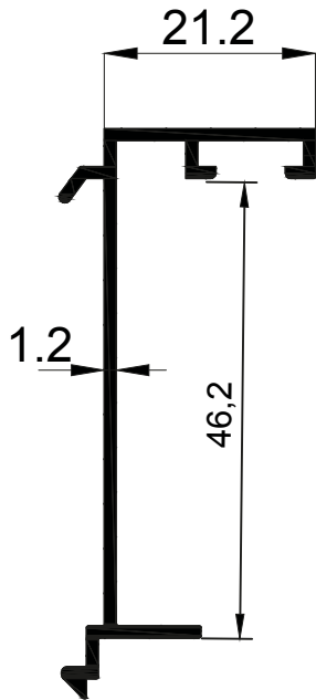
MS3033 0,360 Kg/Mt
