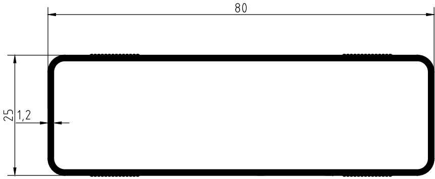
MS8029 0,379 Kg/Mt
