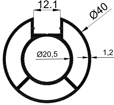
MS1015 0,720 Kg/Mt
