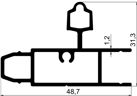
MS5102 0,570 Kg/Mt
