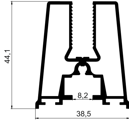
MS5029 0,835 Kg/Mt
