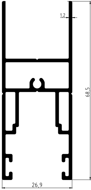
MS5105 0,830 Kg/Mt
