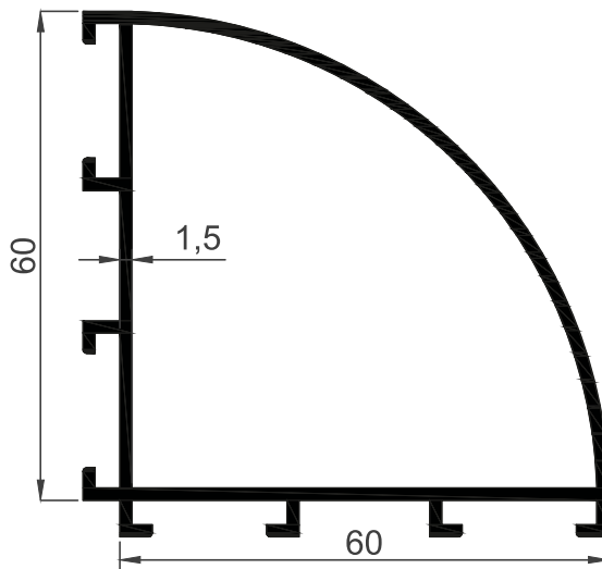
MS3026 1,070 Kg/Mt
