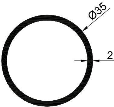
MS1011 0,565 Kg/Mt
