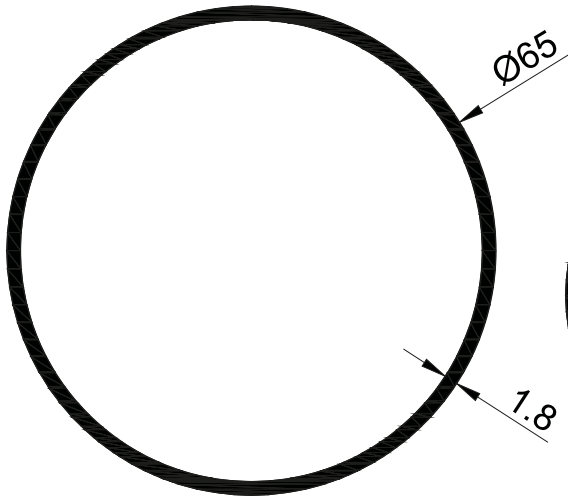
MS1024 0,910 Kg/Mt
