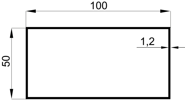
MS2023 0,959 Kg/Mt
