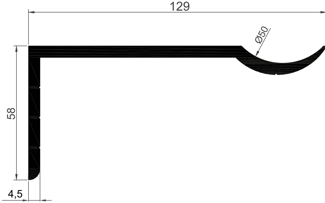
MS7096 2,241 Kg/Mt
