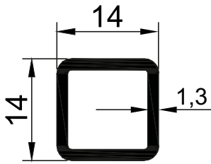
MS1030 0,190 Kg/Mt
