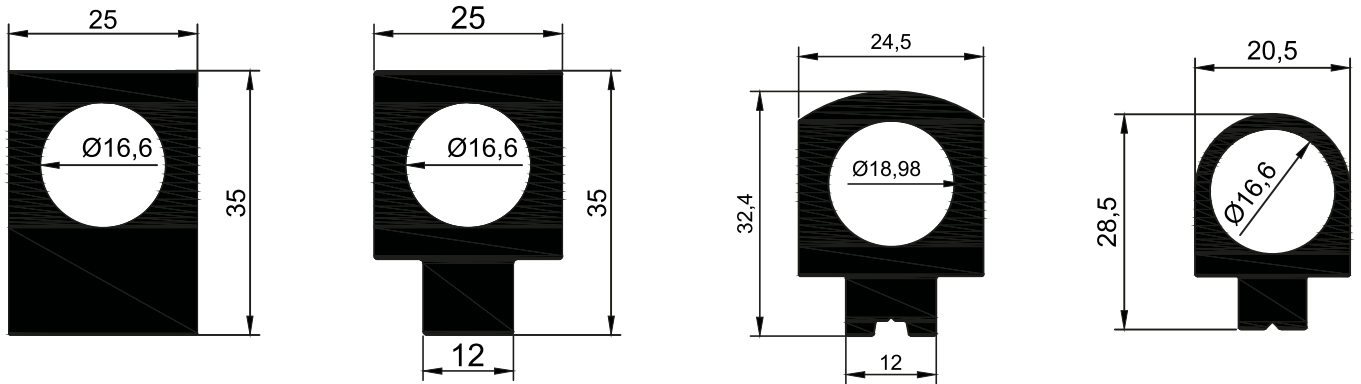
MS7069 1,791 Kg/Mt
