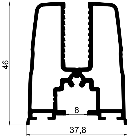
MS5030 0,958 Kg/Mt
