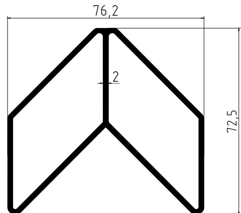
MS5506 0,282 Kg/Mt
